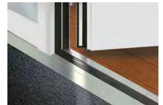
Flachbodenschwelle Spezial mit zusätzlicher Anschlussblende
