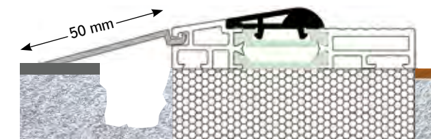
Flachbodenschwelle Spezial mit zusätzlicher Anschlussblende
